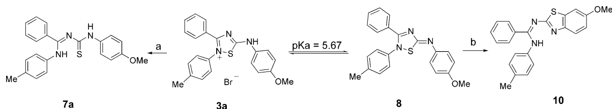
Scheme 2. (a) Dithioerythritol (DTE), dichloromethane; (b) DMSO, 65 °C.
